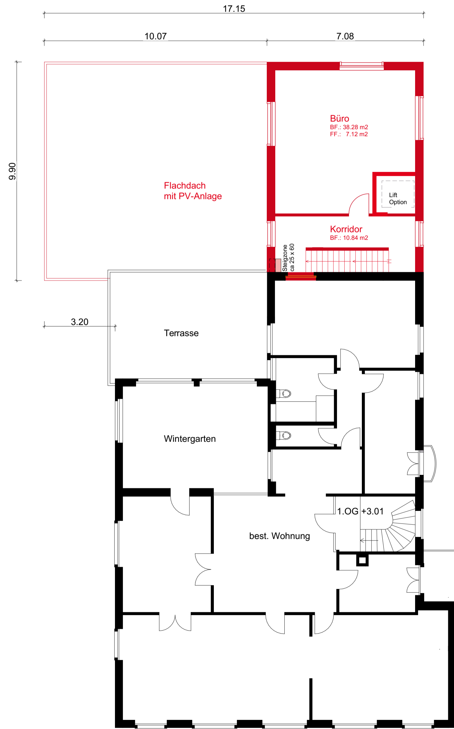
1. Obergeschoss
