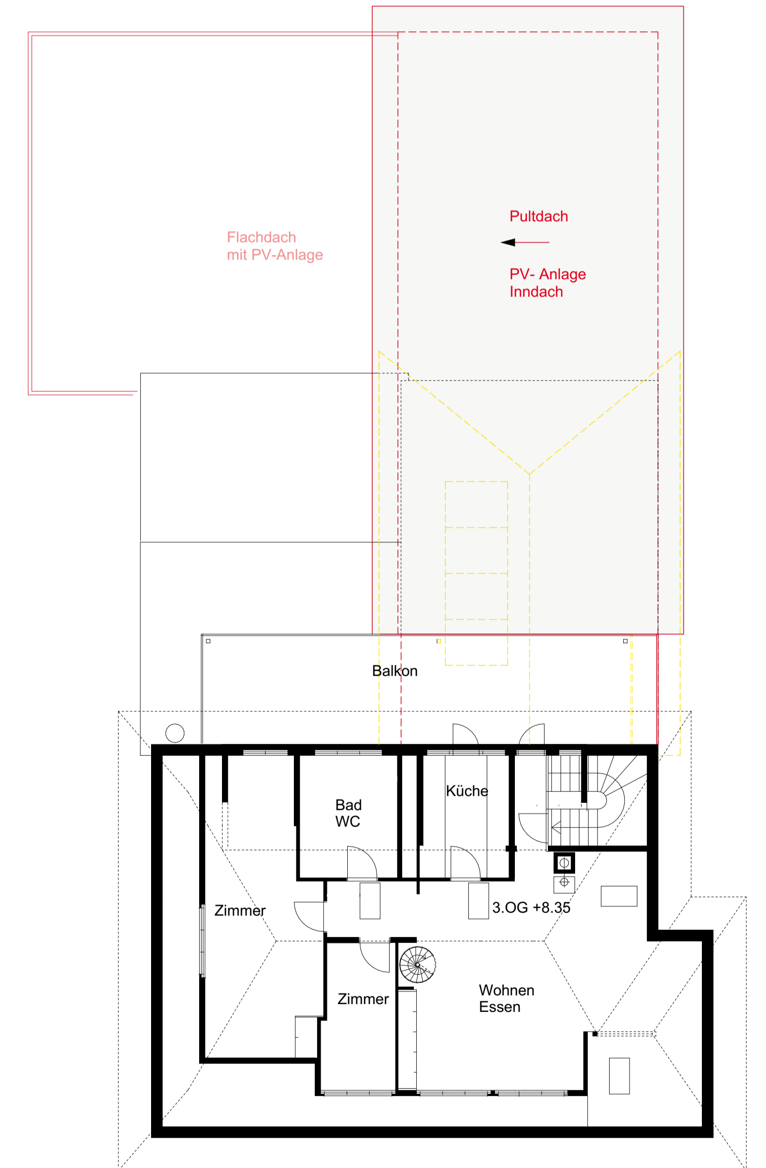
Grundriss 3. Obergeschoss
