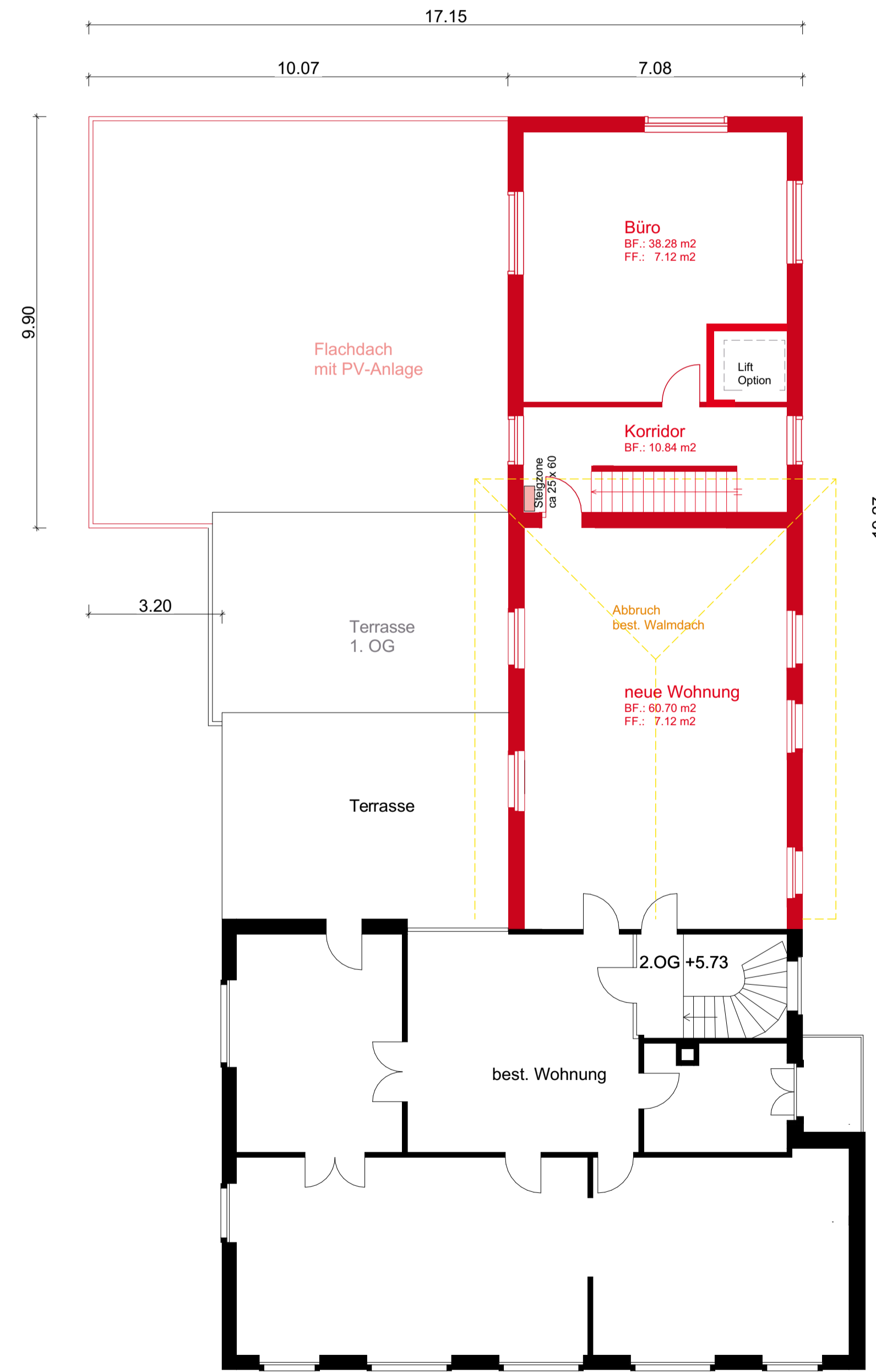
2. Obergeschoss
